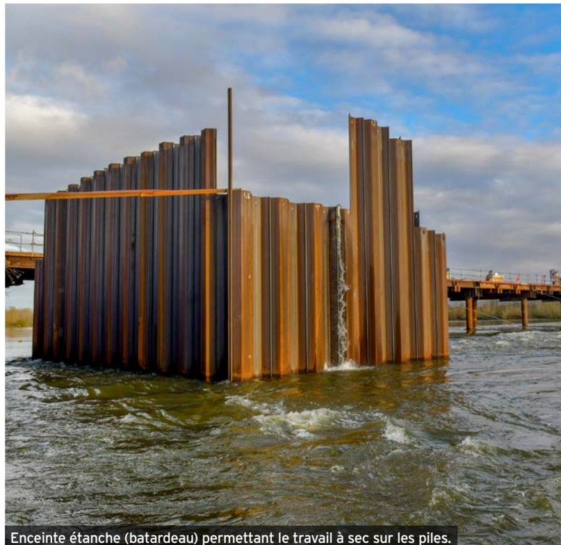
Enceinte étanche (batardeau) permettant le travail à sec sur les piles.
