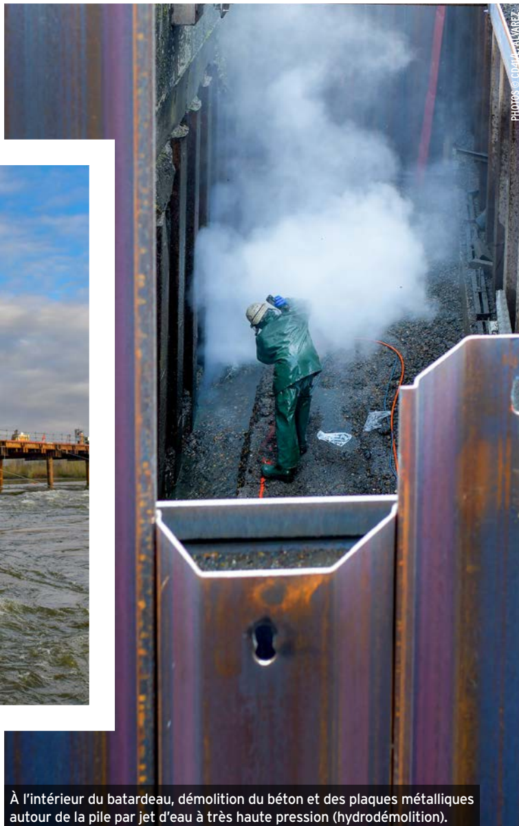
Enceinte étanche (batardeau) permettant le travail à sec sur les piles.
